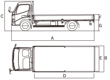
外形図
