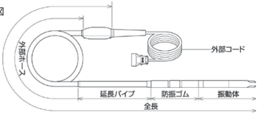
■外形図
