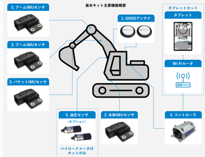
【各種センサーの取り付け】
