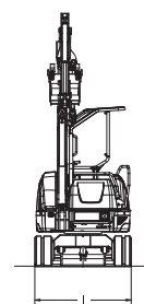
■外形図及び作業範囲図
