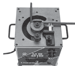
直角曲げカラー使用例
