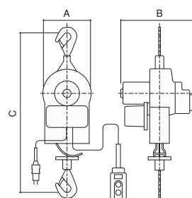
■外形図
