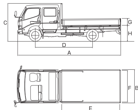
■主要寸法図
