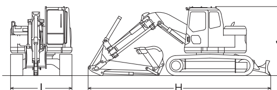
■外形図
