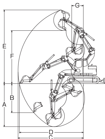
■作業範囲図
