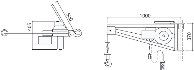
■外形寸法図(単位:)
