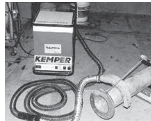
●オプションノズル
