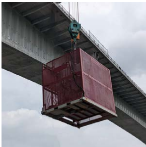
■ 下部ゲージ、昇降フレーム一括吊り ■ レベル出しジャッキ
