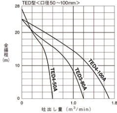
性能曲線 TED型
