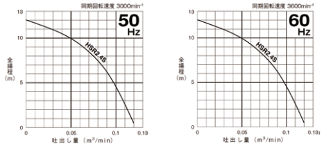
性能曲線
