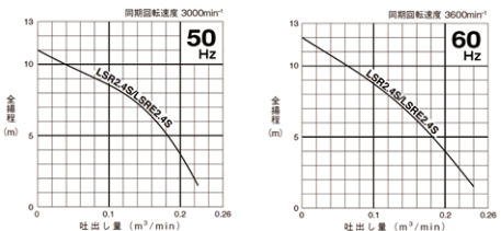
性能曲線
