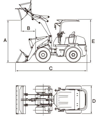
外形図
