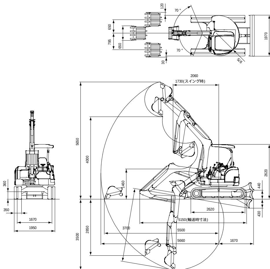
キャノピ仕様外形図
