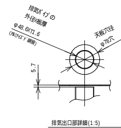
排気出口部詳細(1:5)
