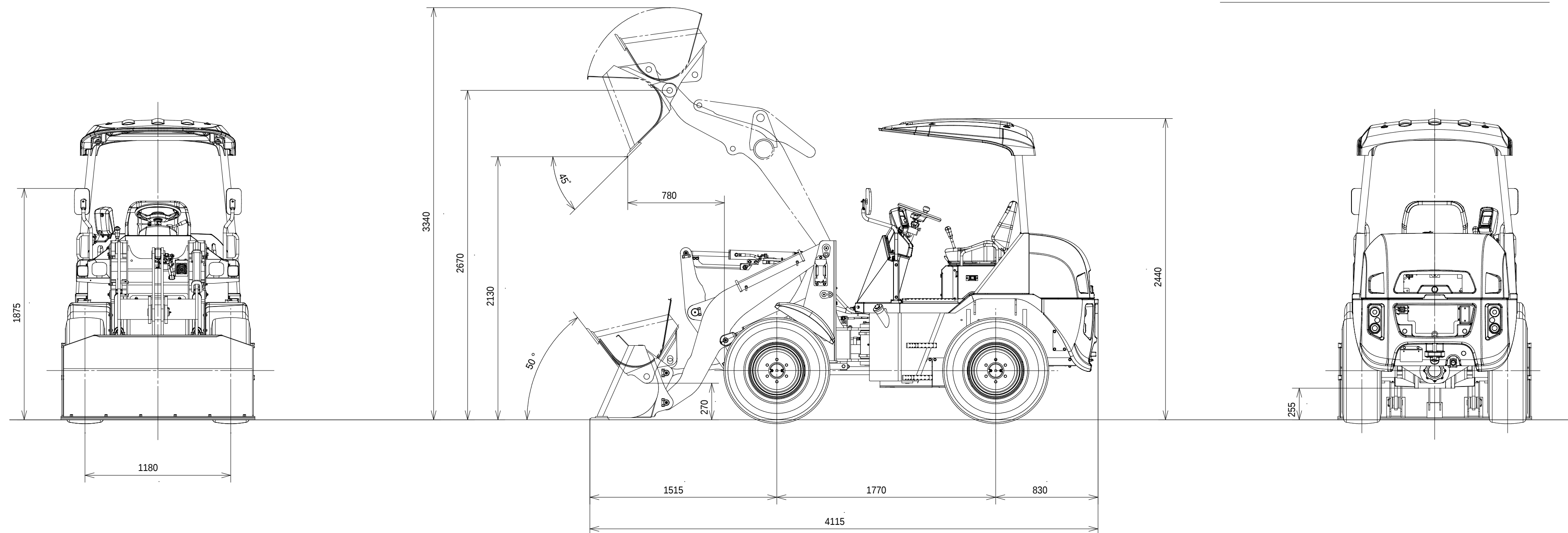
V3-7-P 外形図
