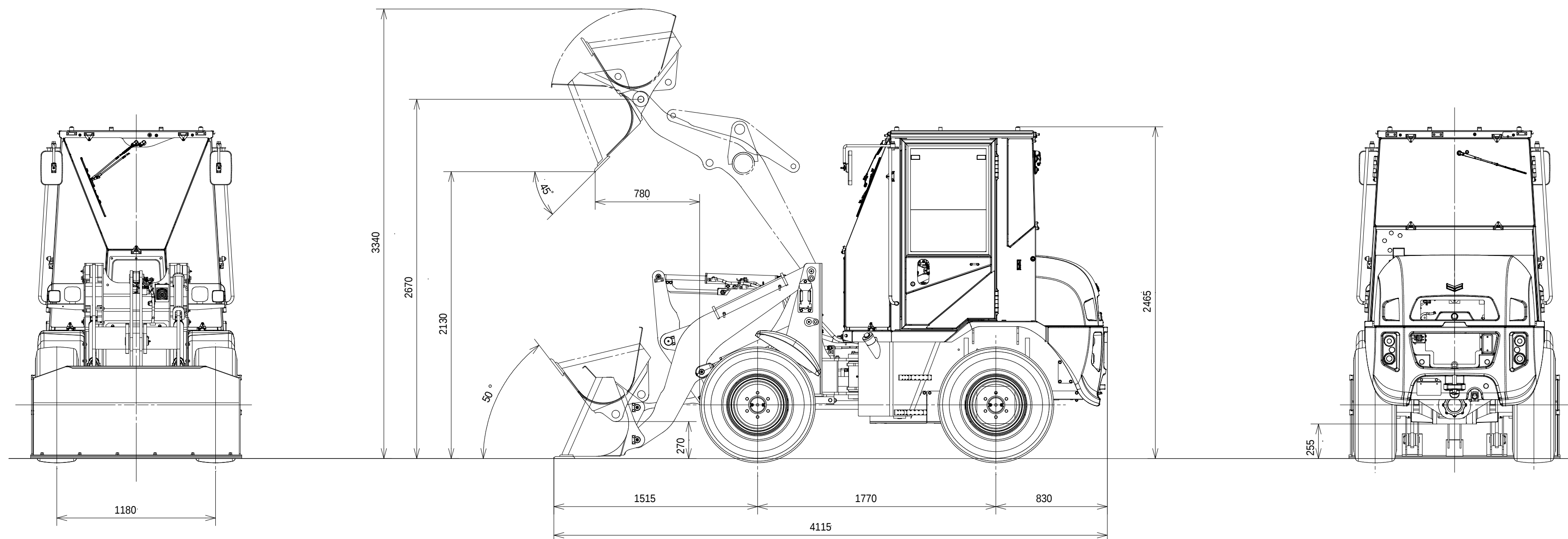
V3-7-C 外形図
