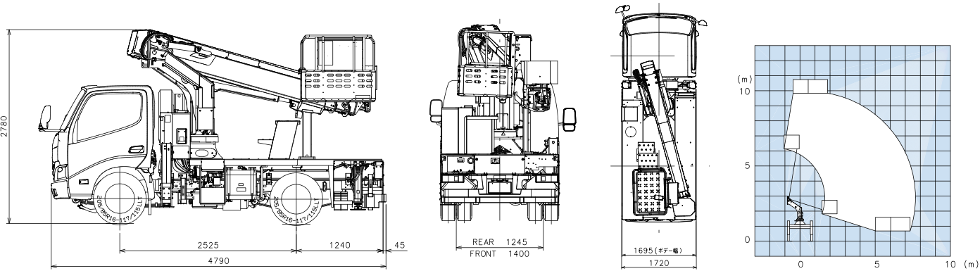
※車両寸法図における単位はmmです。 ※車両寸法は架装シャシーにより異なります。
