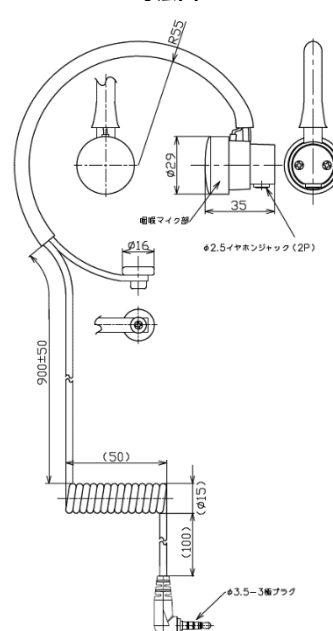
寸法図
