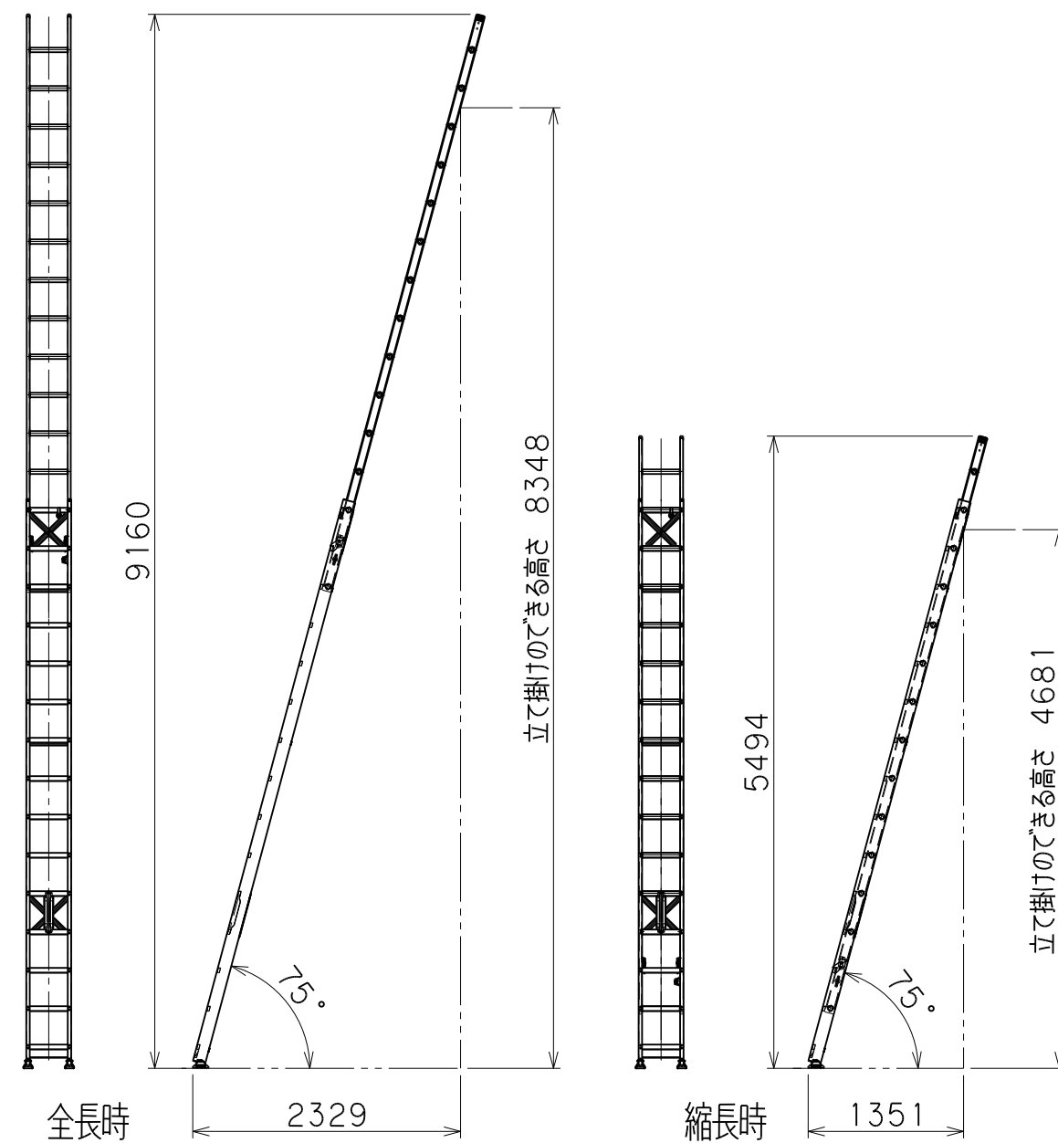
立て掛け寸法図 (1/60)
