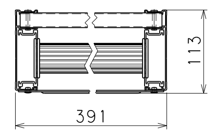
A-A断面図 (1/5)
